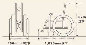
⚠ 収納できる車いすの寸法 (折り畳み時)
