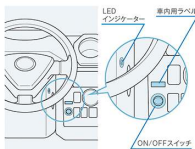
キーレスエントリー車
